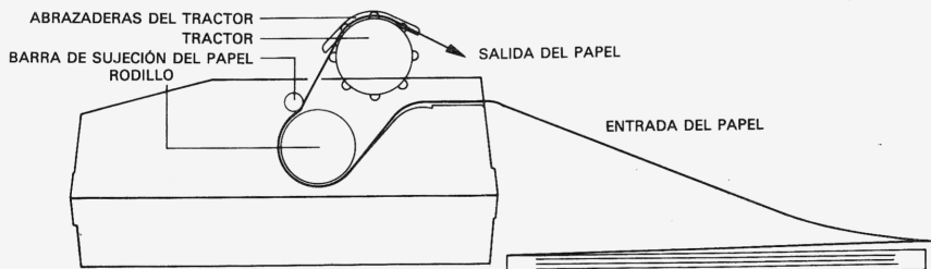
Trayectoria de alimentación de papel continuo
