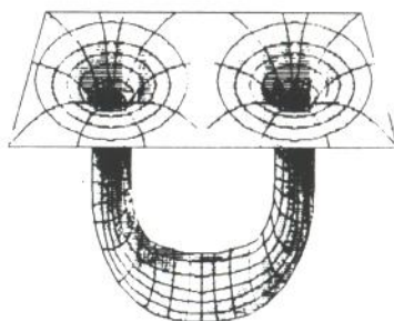
fig 3 : l'espace-temps, tel que l'a démontré Rolf
