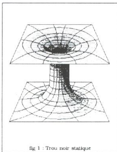
fig 1 : Trou noir statique
