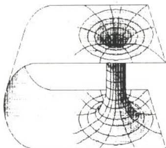
fig 2 : l'espace-temps imaginé par Einstein et Rosen
